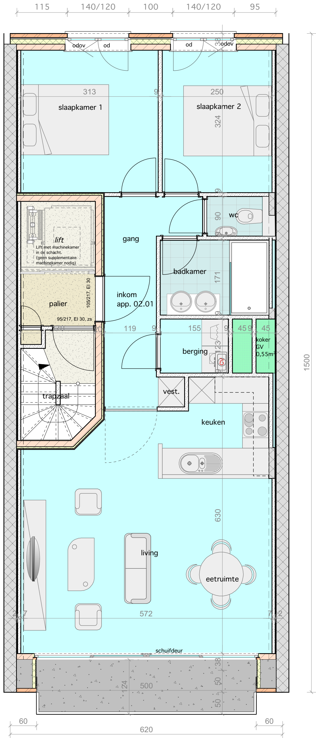
Verdieping 2
